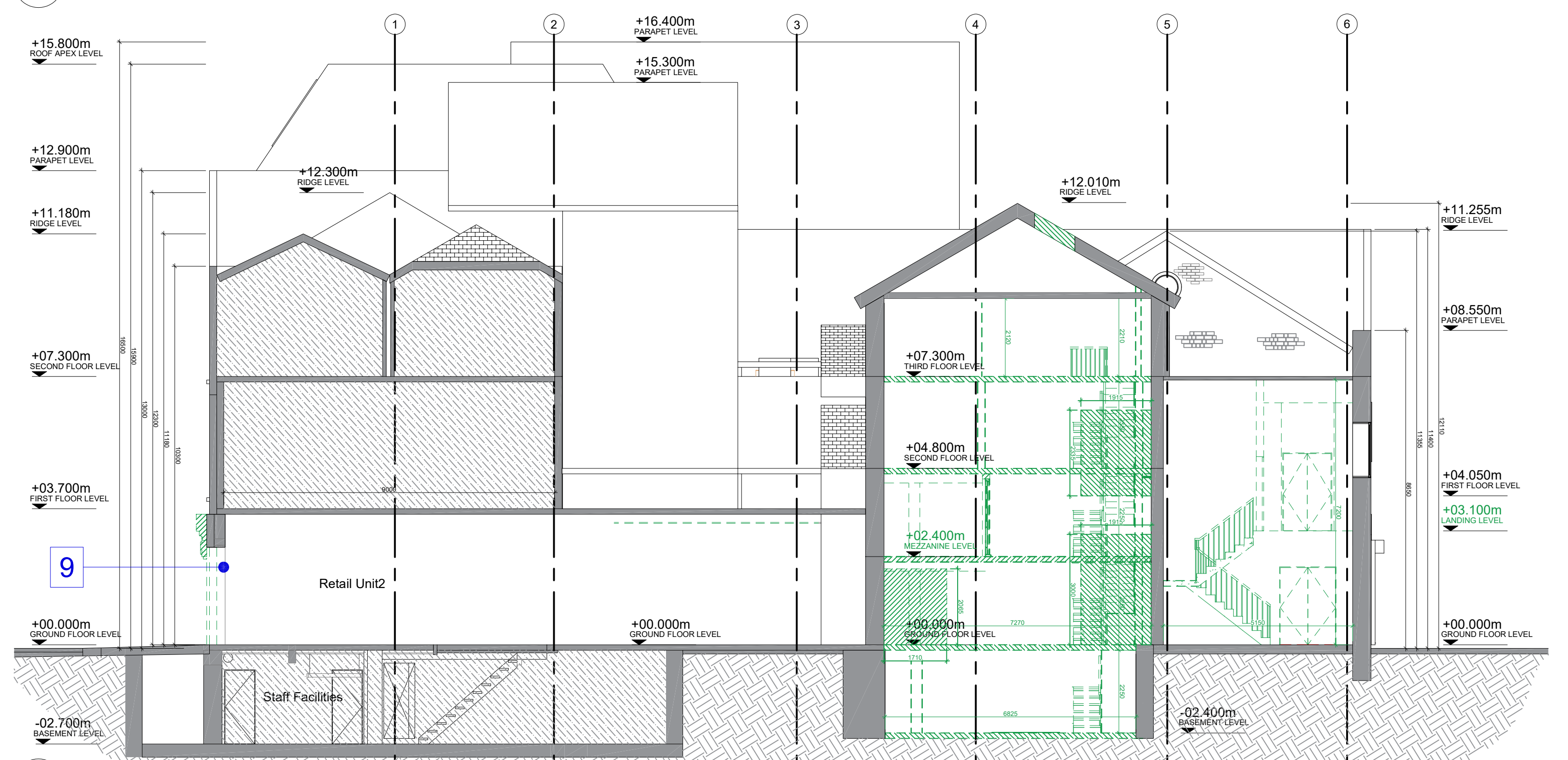
SECTION B-B SCALE: 1:100
