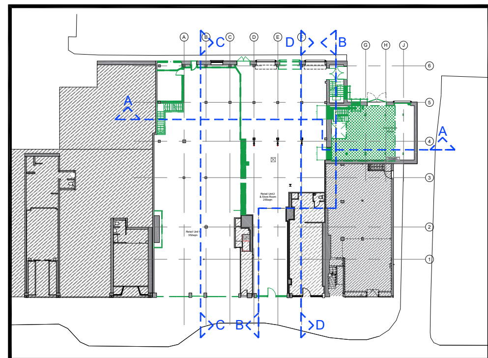
GFL_KEYPLAN SCALE: NTS
